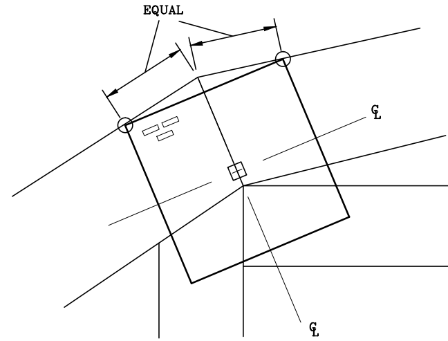
MITRE JOINT
